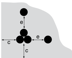
Figure n° 24 : distances minimales des armatures aux coffrages, et entre elles, (en mm) permettant la transmission des forces d'adhérence et un bétonnage correct suivant la norme NF EN 1992-1-1.
