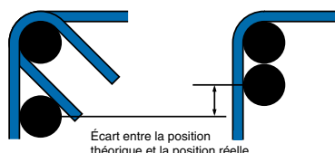
Figure n° 35 : fermeture des cadres, difficulté de mise en place de barres superposées.
